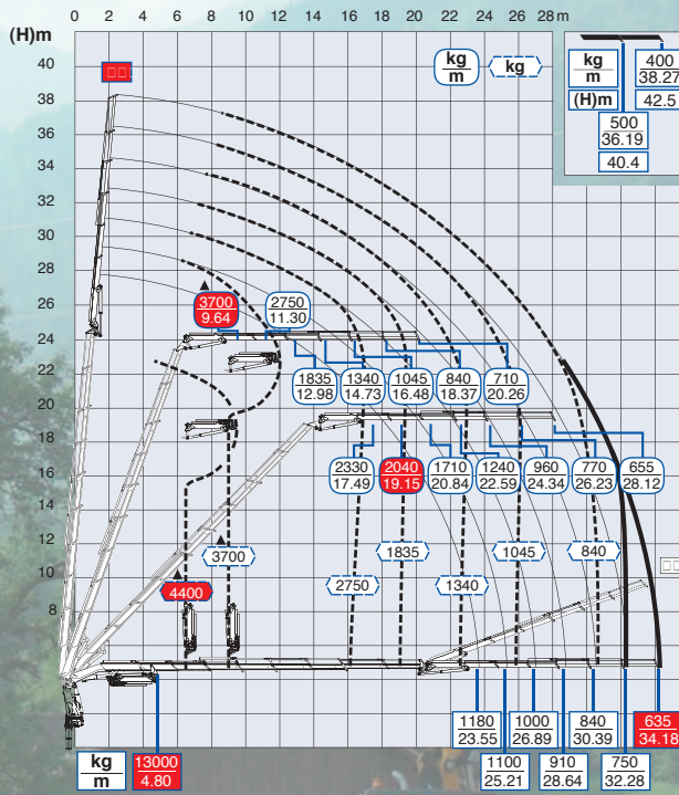
Leistungsdaten unseres 41-Meter-LKW-Krans
